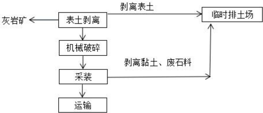
图4-4 非爆破开采工艺流程图
