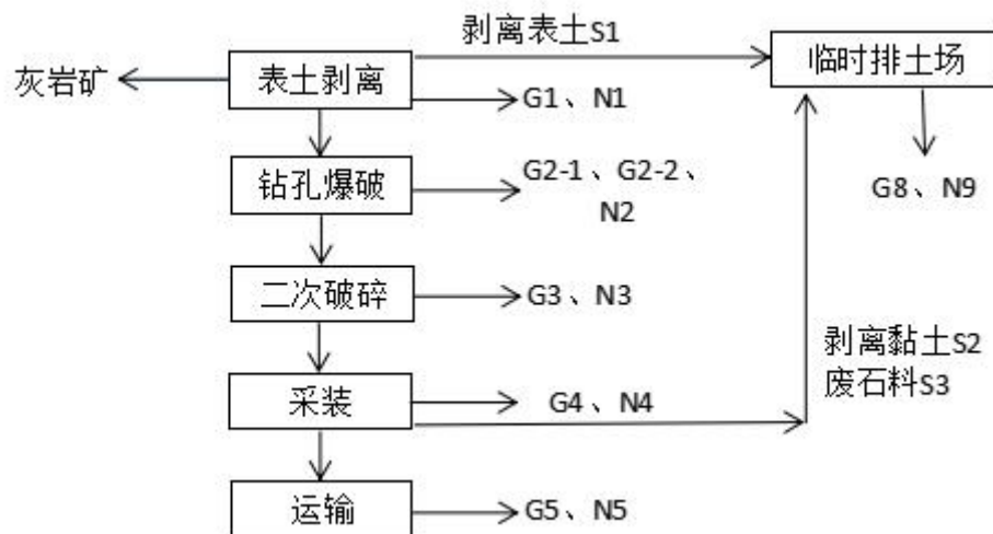
图4-2 项目采矿工艺流程及产污节点图
