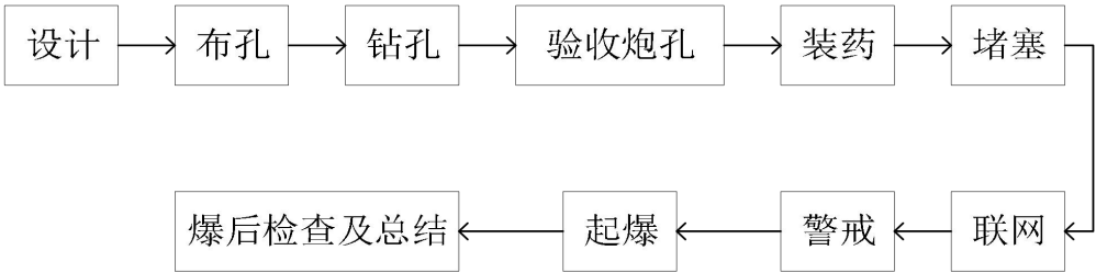
图4-3 采矿爆破工艺流程图
